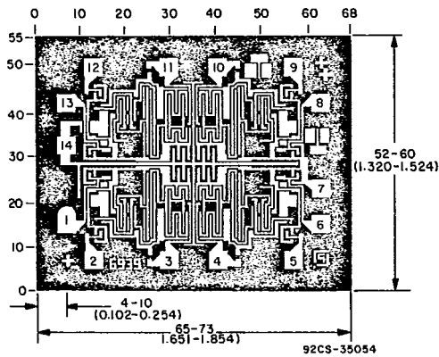
CD4001B
