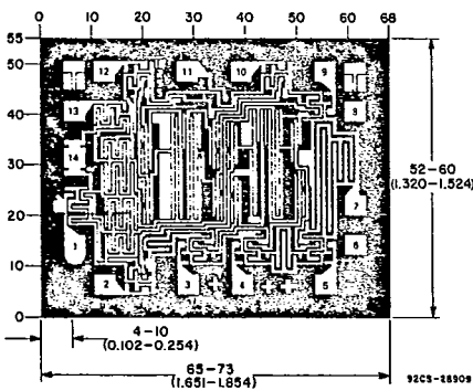
CD4002B
