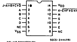
CD4002B
