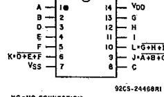
CD4025B
