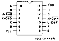
CD4001B
